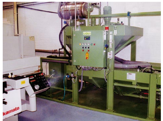
Disc-O-Filter® Typ 250
